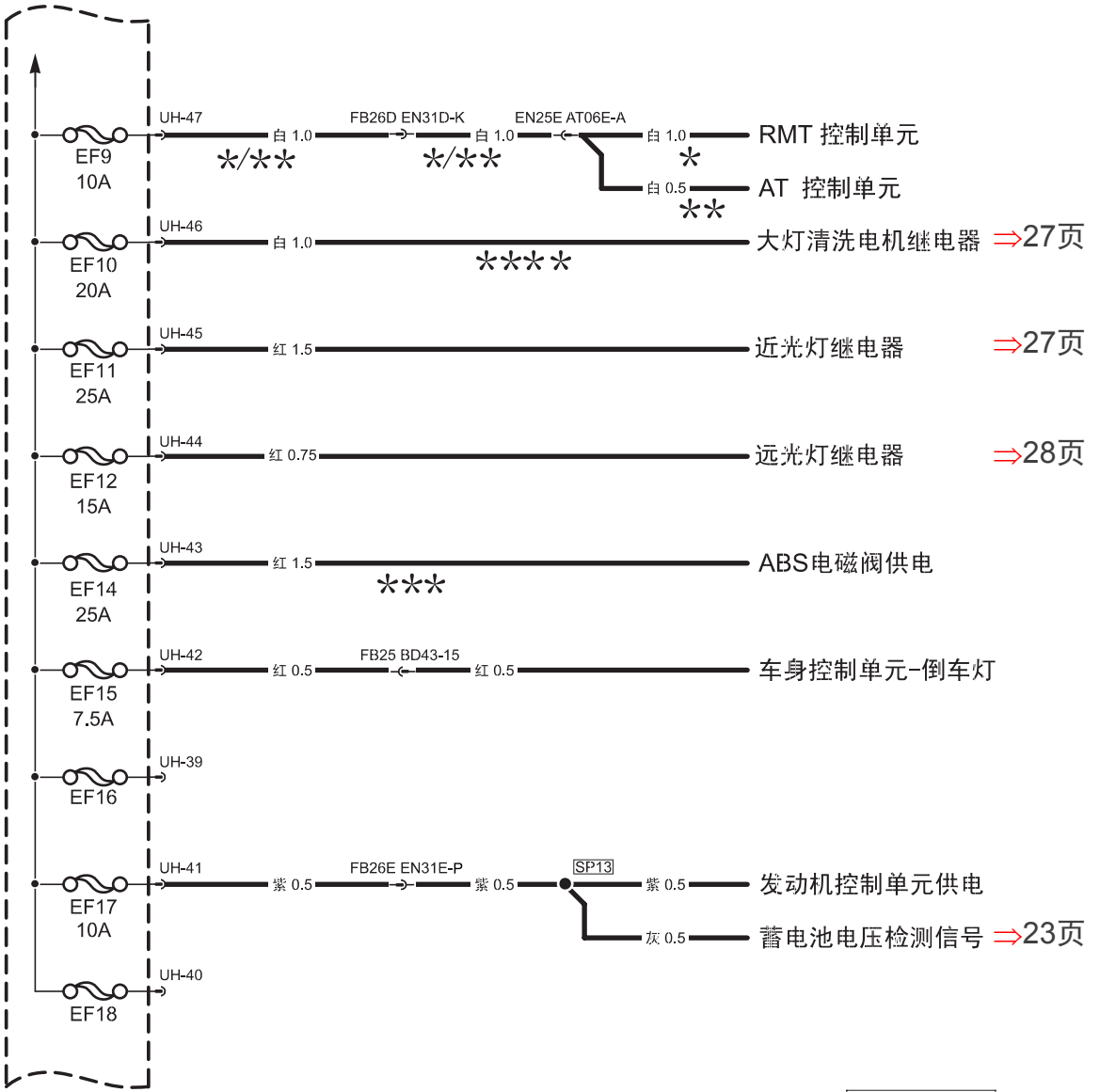
前舱继电器盒
